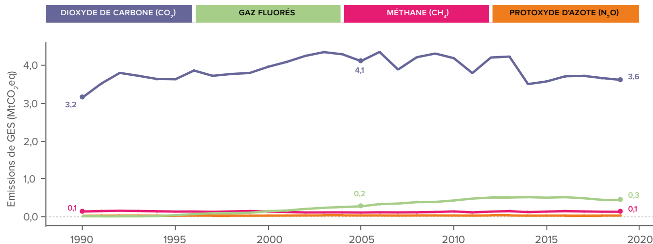
Résidentiel - Évolution des émissions de GES.
