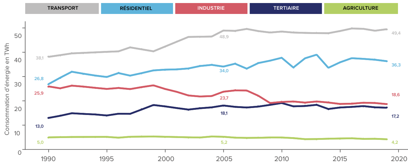
Évolution des consommations d'énergie finale par secteur (hors consommations non sectorisées) de 1990 à 2019.
