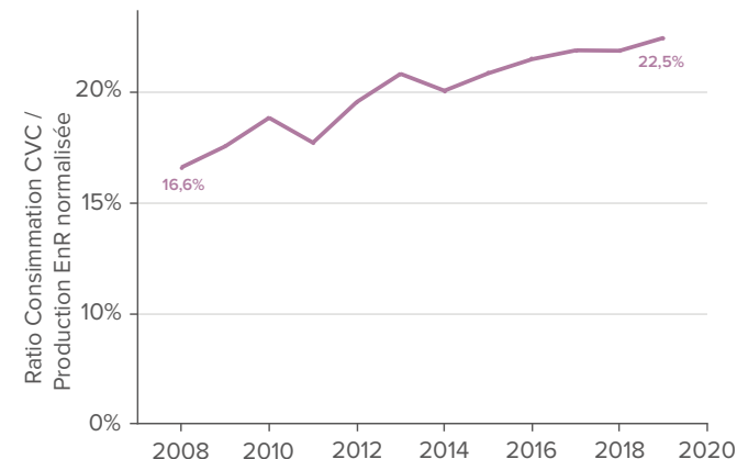
Évolution de la part d'énergie renouvelable dans la consommation d'énergie finale de 2008 à 2019.
