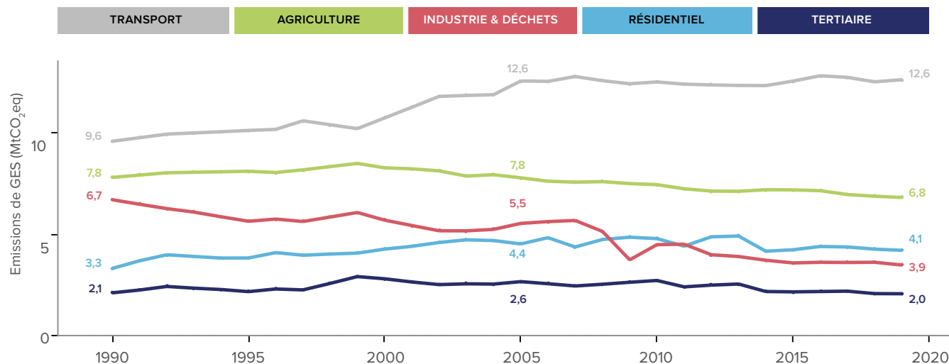
Évolution des émissions de GES par secteurs de 1990 à 2019.
