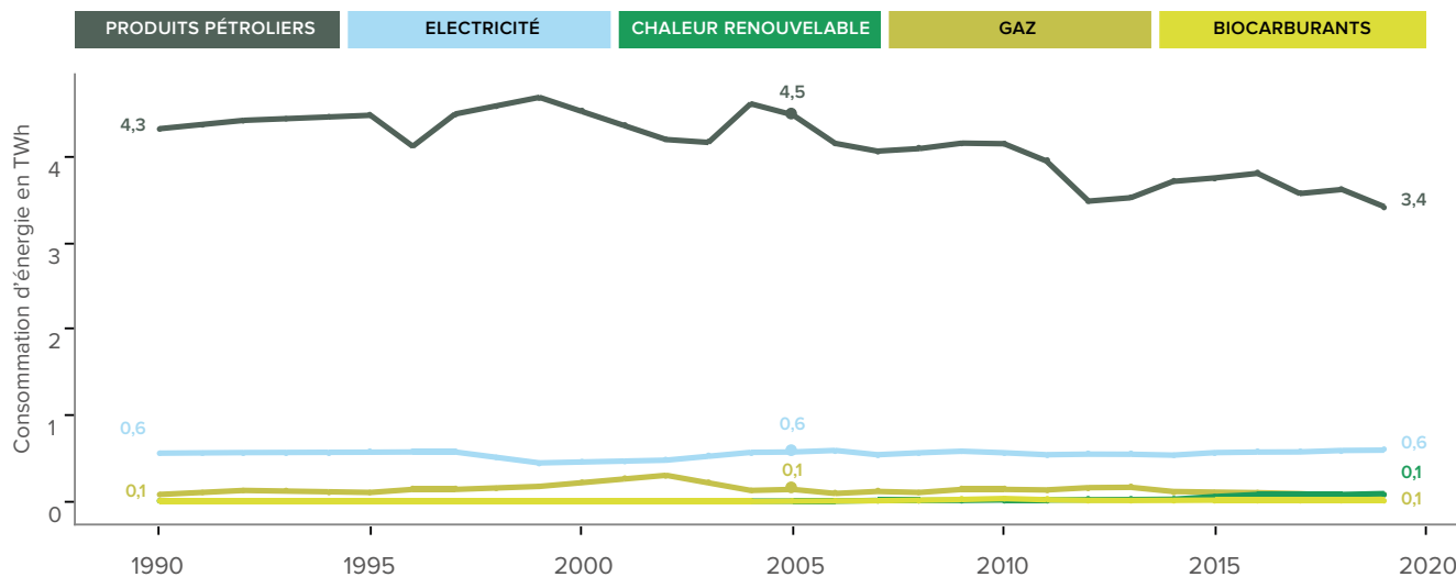
Agriculture - Évolution des consommations.
