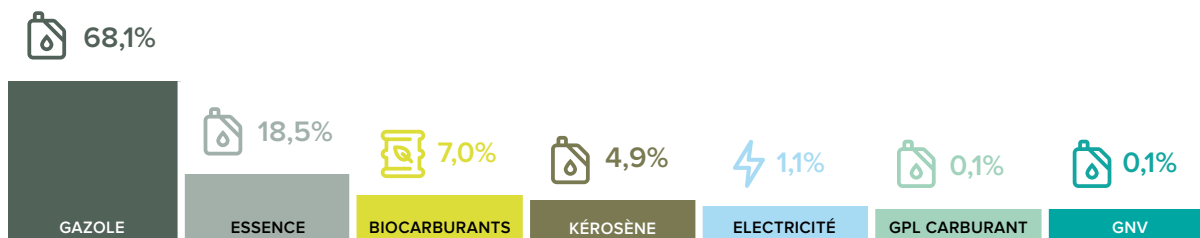
Transports - État des lieux du mix énergétique en 2019.
