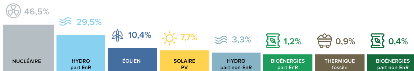
Mix de production électrique en 2020.
