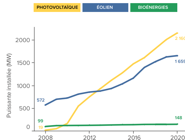
Évolution des capacités installées d'EnR électrique (hors hydroélectricité).
