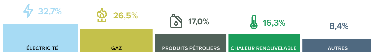
Industrie et déchets - Etat des lieux du mix énergétique en 2019.
