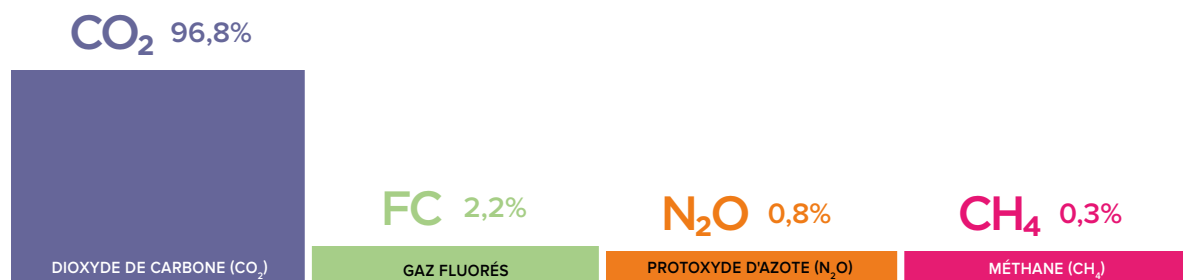
Transports – Zoom sur la répartition des émissions de GES en 2019.
