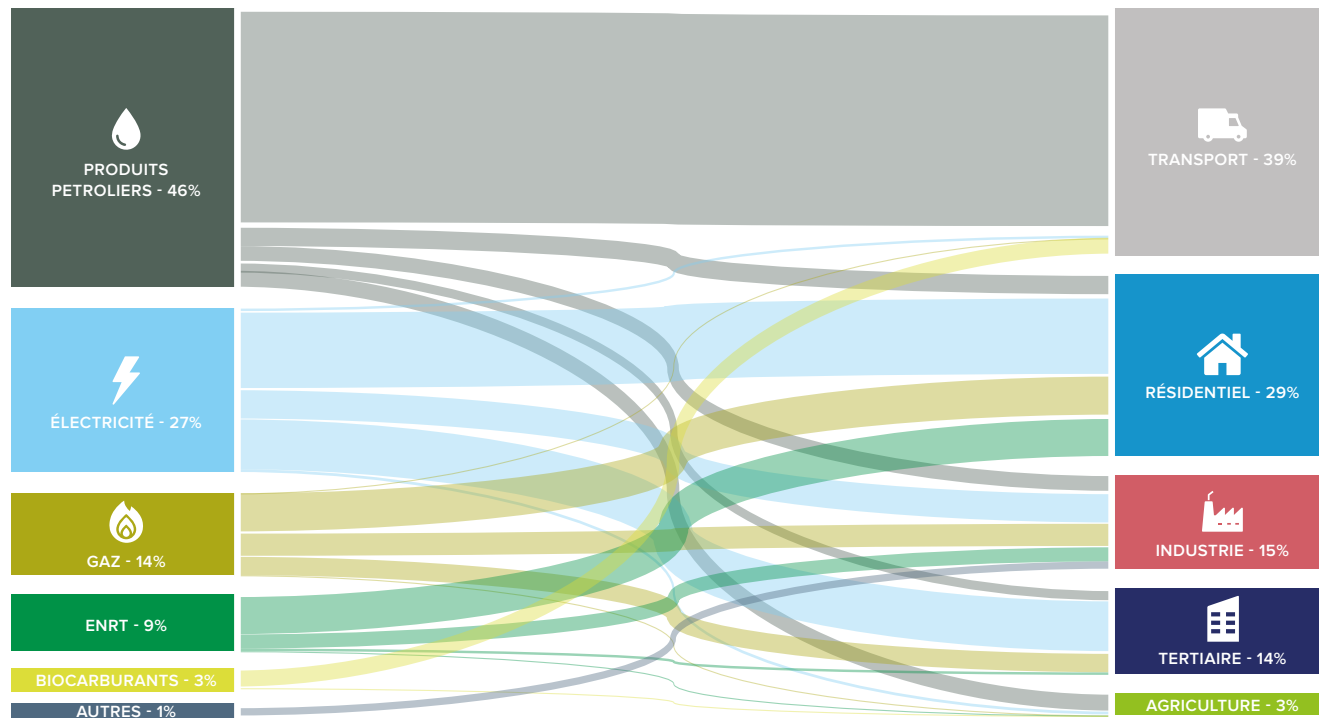
Consommation d'énergie finale en 2019.
