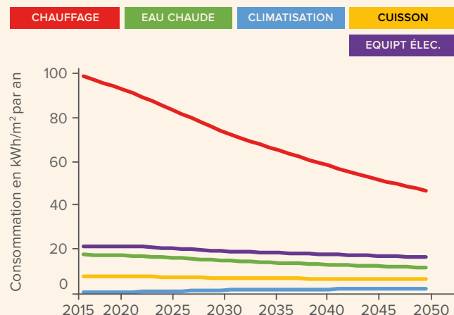
Scénario REPOS Résidentiel. Évolution 2015-2050 des consommations par usages.
