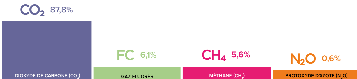
Industrie et déchets - Zoom sur la répartition des émissions de GES en 2019.
