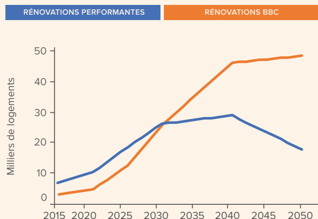
Scénario REPOS Résidentiel. Rythme annuel de rénovation.
