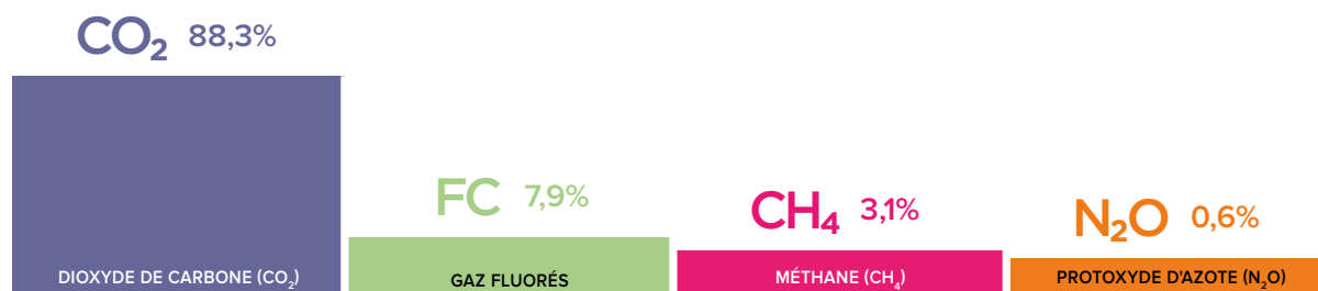
Résidentiel - Zoom sur la répartition des émissions de GES en 2019.
