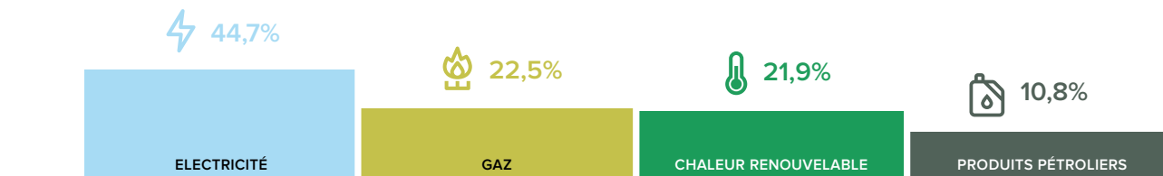
Résidentiel - Etat des lieux du mix énergétique en 2019.
