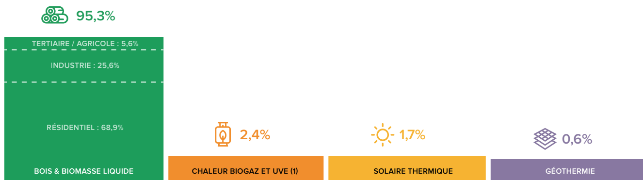
Mix de production de chaleur renouvelable en 2020.
