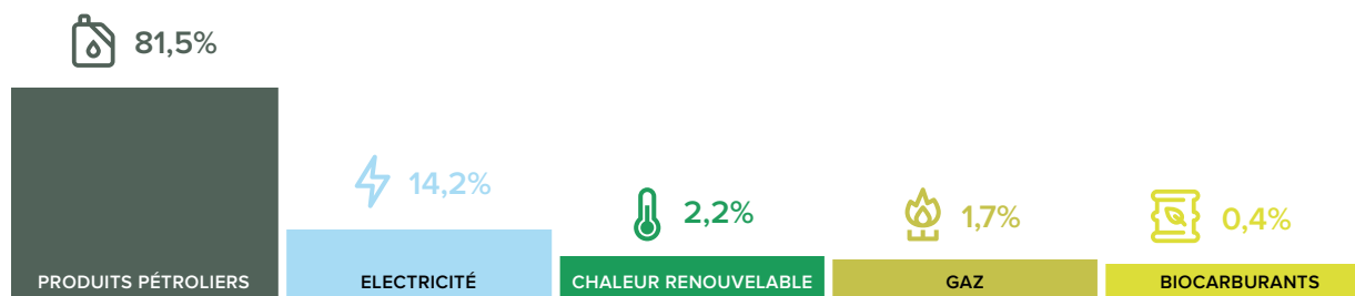
Agriculture - Etat des lieux du mix énergétique en 2019.
