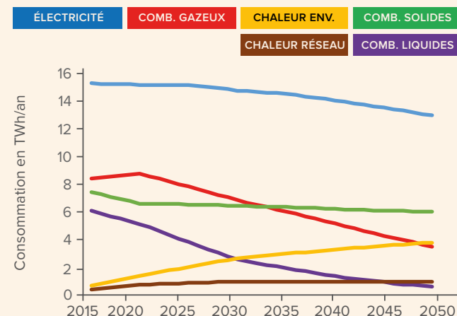
Scénario REPOS Résidentiel. Évolution 2015-2050 des consommations par vecteurs énergétiques (en TWh).
