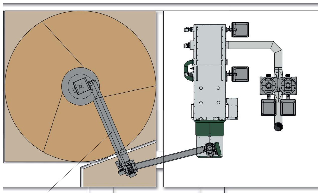
Dessilleur avec entraînement indépendant
