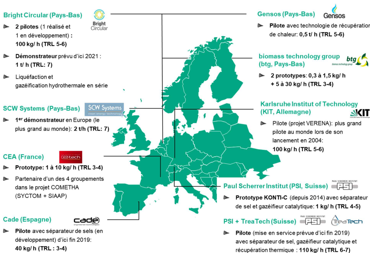
Figure 2 – Principaux développements technologiques sur la gazéification hydrothermale en Europe
