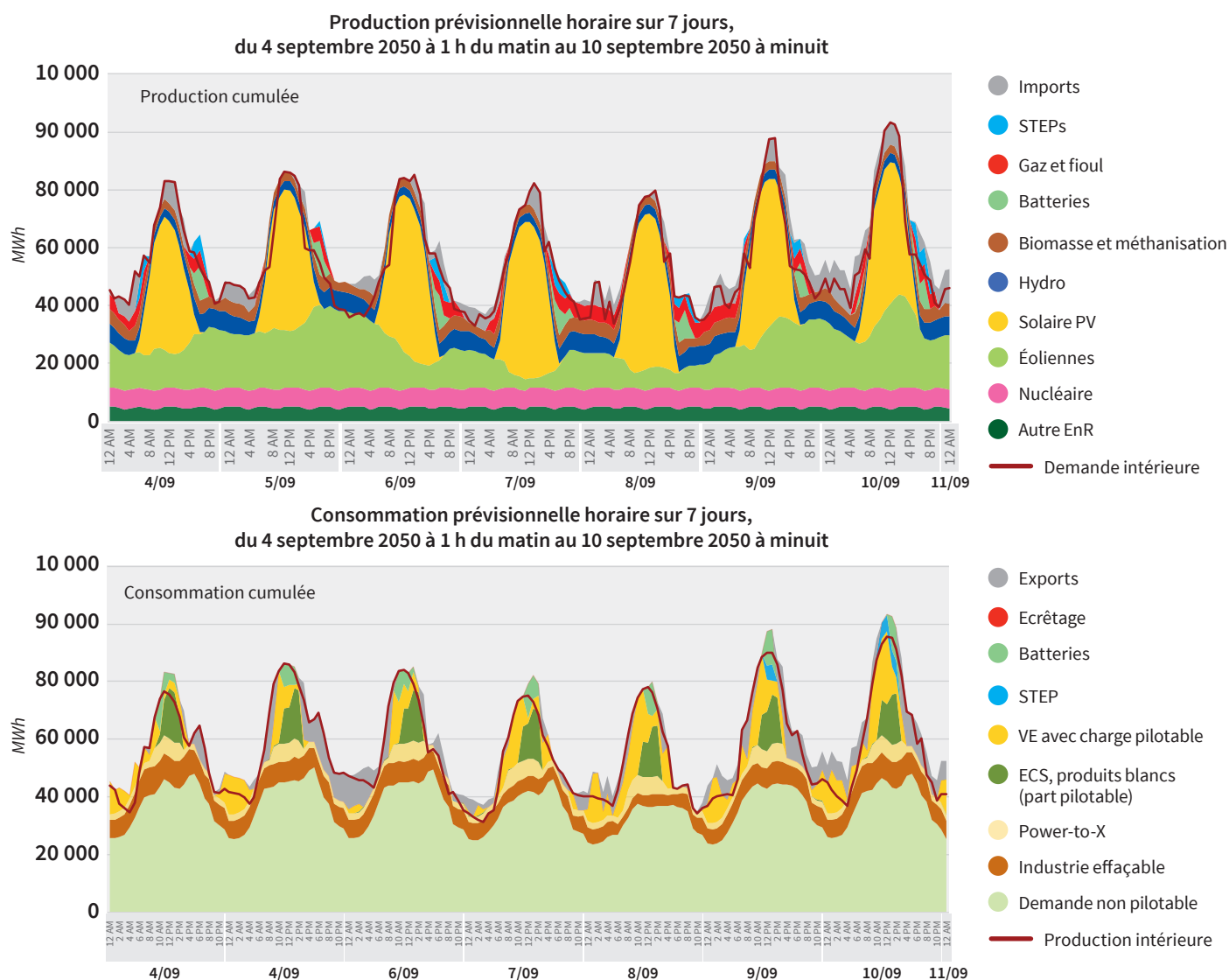
FIGURE 7 : EXEMPLE DE RÉSULTAT DU MODÈLE SUR UNE SEMAINE DE SEPTEMBRE 2050 (EN HAUT, L'APPEL DES DIFFÉRENTS MOYENS DE PRODUCTION ; EN BAS, LA DÉCOMPOSITION DE LA DEMANDE) (21)
