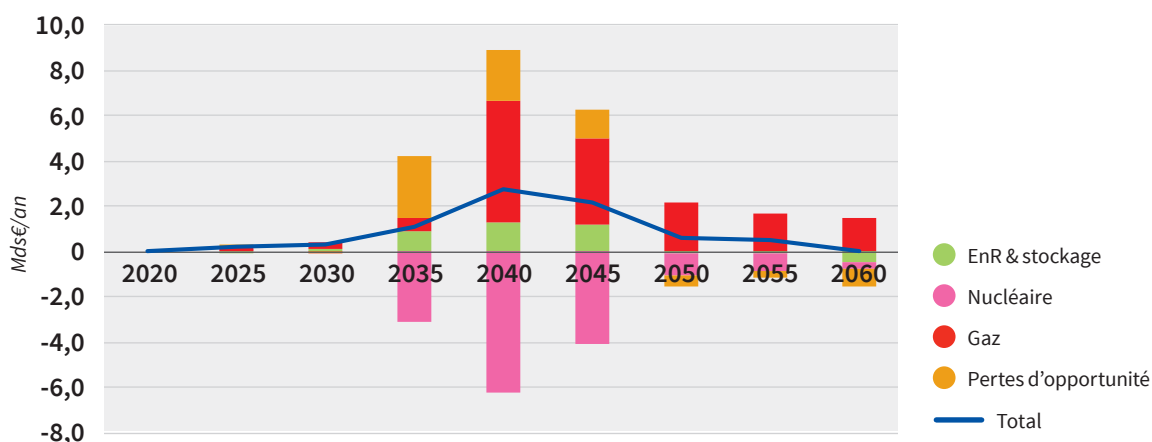
FIGURE 14 : COÛTS SUPPLÉMENTAIRES DU SCÉNARIO « FERMETURE DES CENTRALES NUCLÉAIRES À 50 ANS » PAR RAPPORT À LA TRAJECTOIRE DE RÉFÉRENCE
