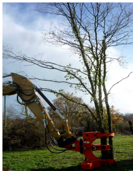
Tête d'abattage
